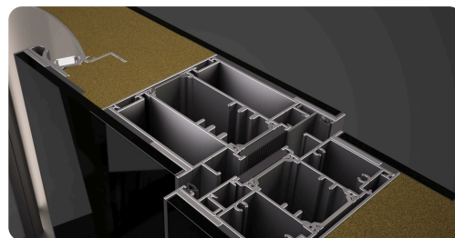
Τομή προφίλ pivot / aller-retour
