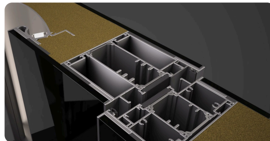
Τομή pivot / aller-retour — θερμοδιακοπή πολυαμιδίου 32 mm
